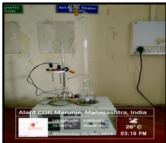
Karl Fischer Titration Apparatus
